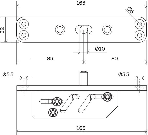
TOP PIVOT
