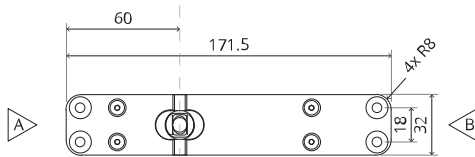
Vista dall'alto
