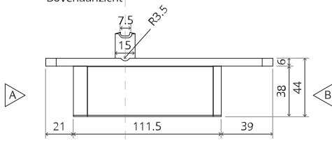
Vooraanzicht
